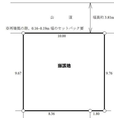
■ 区画参考図
